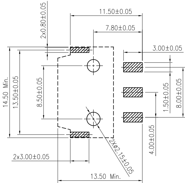
P.C.B. Layout
