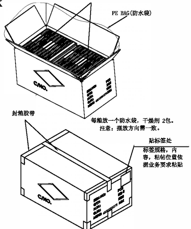
2叠产品装1箱, 3120PCS/箱。干燥剂 (2包)
