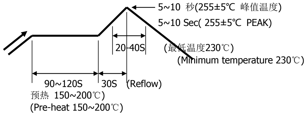
温度条件曲线图/ 基板上温度
