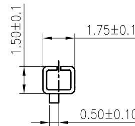
SECTION D-D
