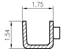
SECTION D-D
